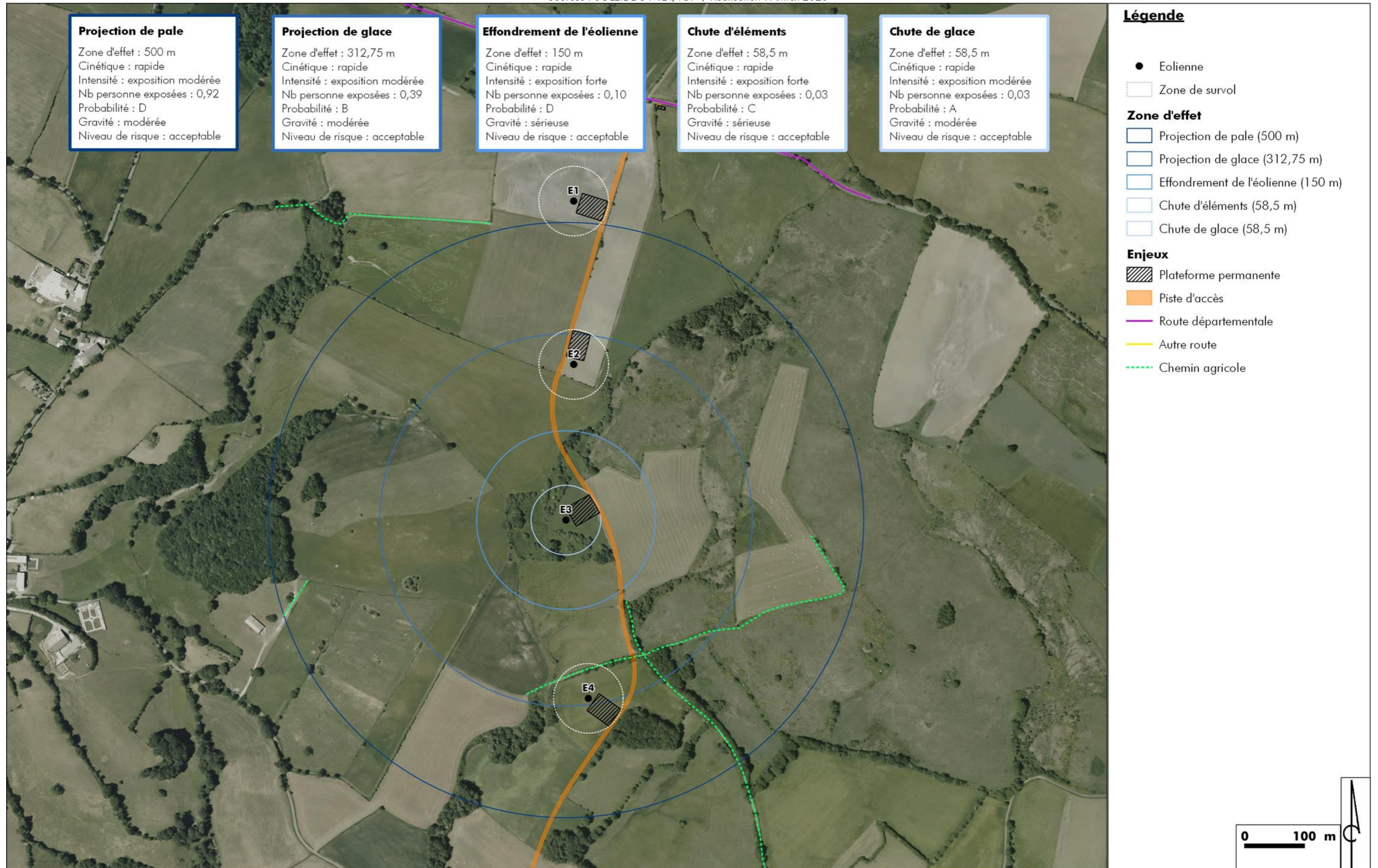
Illustration 9 : Carte de synthèse des risques pour l'éolienne E3
