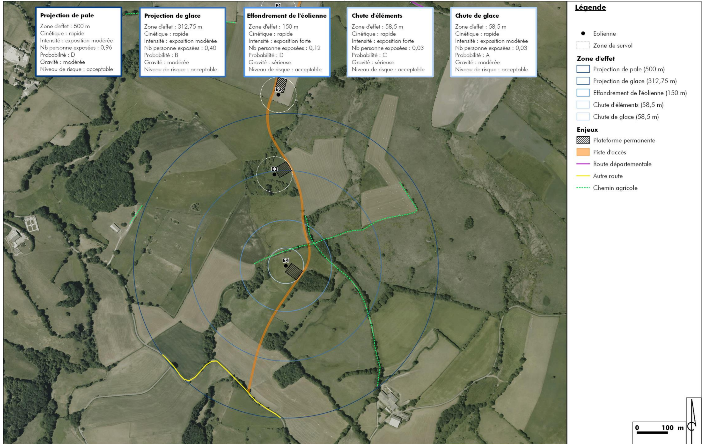
Illustration 10 : Carte de synthèse des risques pour l'éolienne E4
