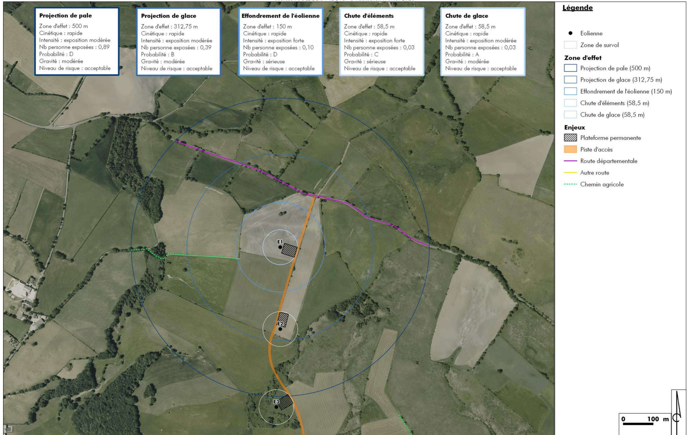
Illustration 7 : Carte de synthèse des risques pour l'éolienne E1
